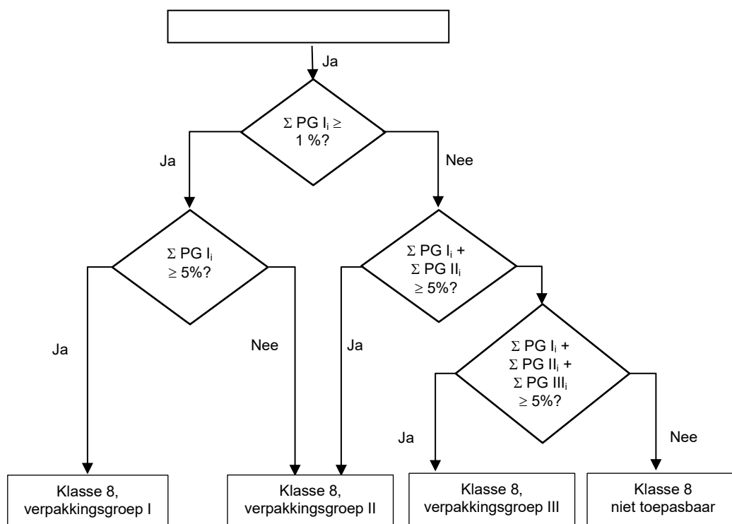
Figuur 2.2.8.1.6.3: Berekeningsmethode
